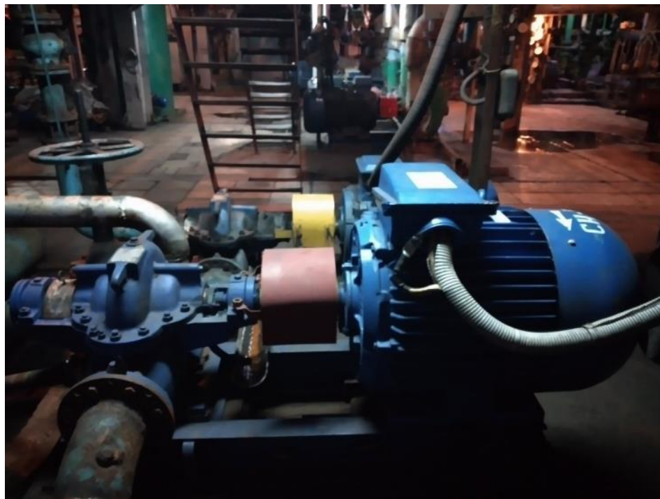
НАСОСНЫЙ АГРЕГАТ 4Д 200-90 НА КОТЕЛЬНУЮ «ЦЕНТРАЛЬНАЯ» ВОСТОЧНЫЙ ЛУЧ
