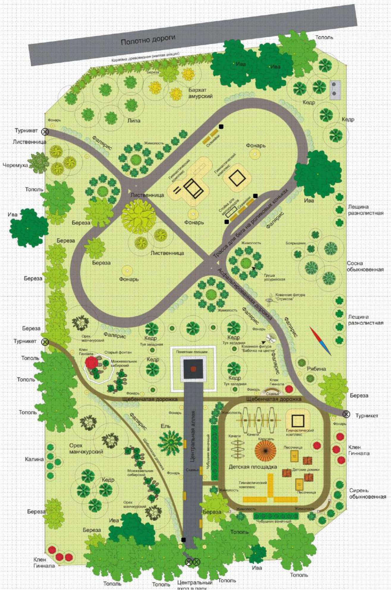
Генплан благоустройства сквера по ул. Слюдянских Красногвардейцев в г.Слюдянка Масштаб 1:400 (клетка масштабной сетки соответствует 1 метру)
