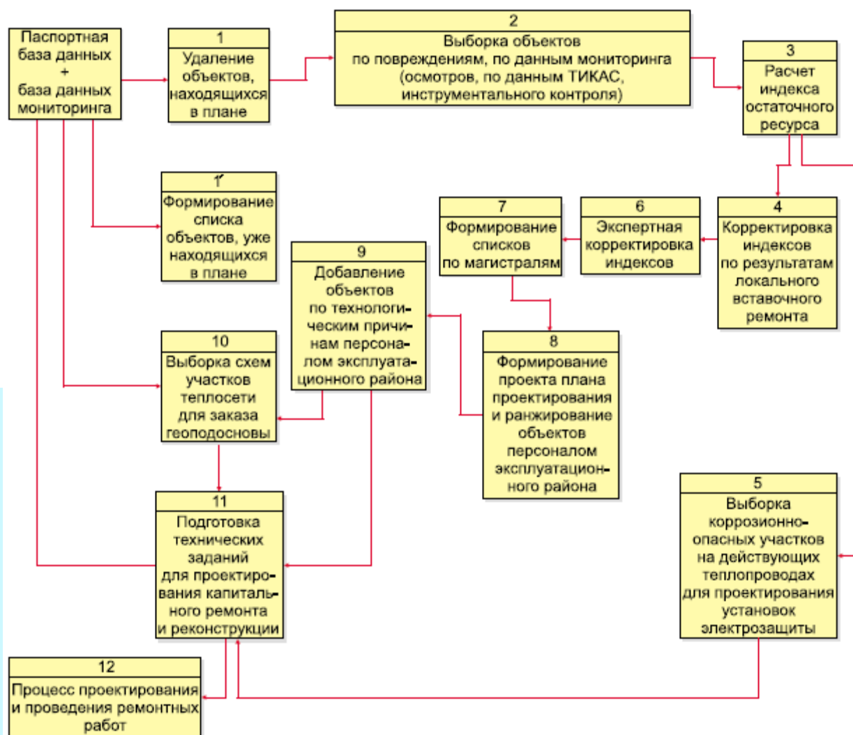
Рисунок 1.7 – Схема формирования плана проектирования и переключок
