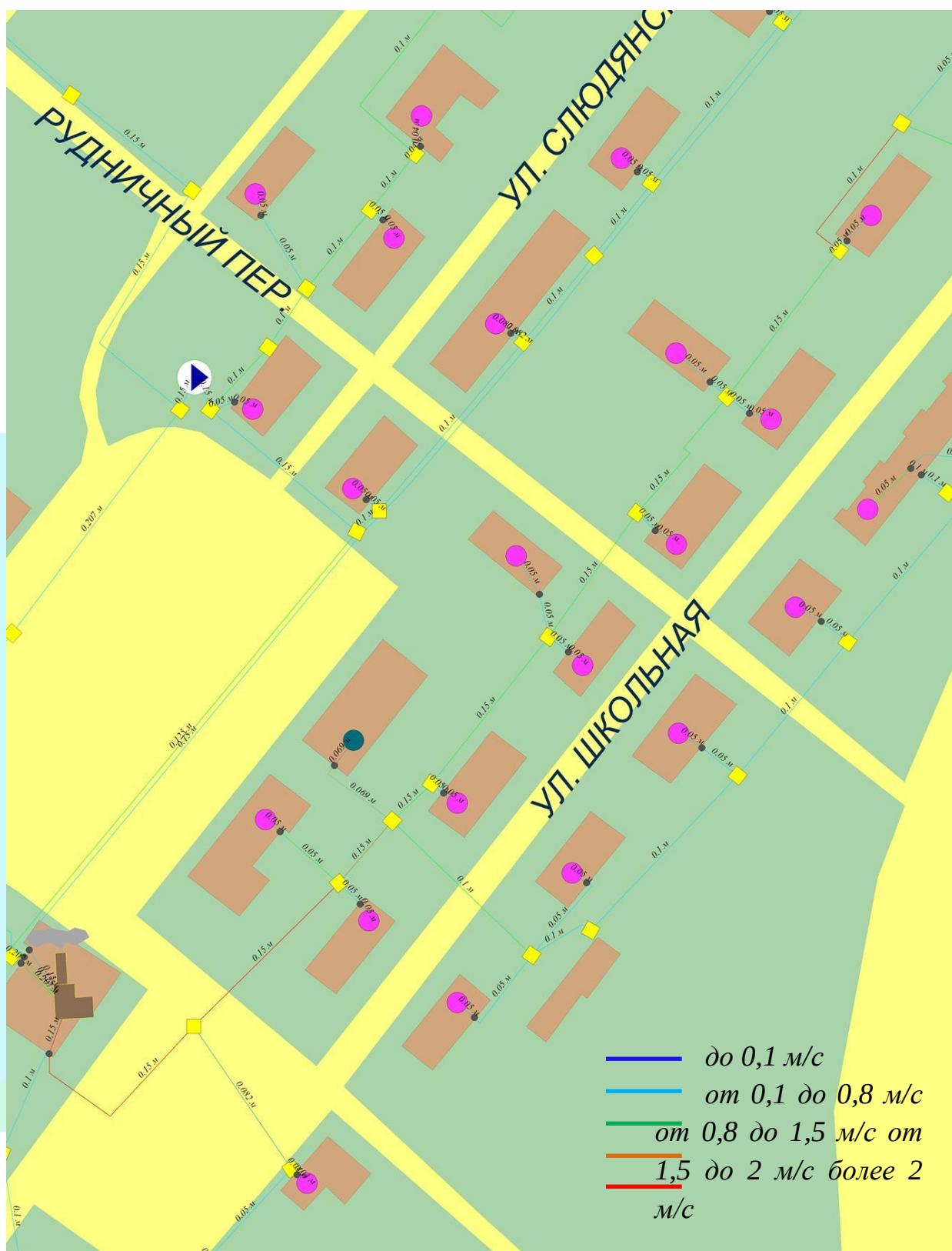
Рис.3.11 - Скорости теплоносителя по участкам теплосети от котельной Рудо
