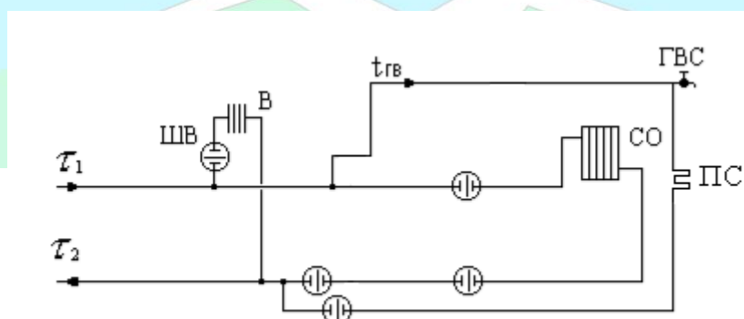
Рисунок 1.5 – Потребитель с открытым водоразбором и циркуляционной линией для микрорайона «СМП»
