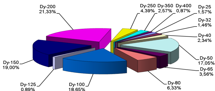
Рисунок 1.3 – Доля тепловых сетей по диаметрам
