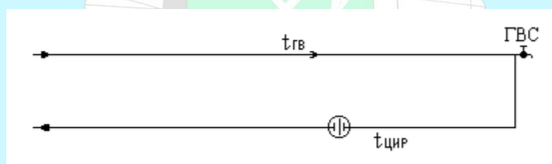
Рисунок 1.5 – Потребитель с открытым водоразбором и циркуляционной линией для микрорайона «СМП»
