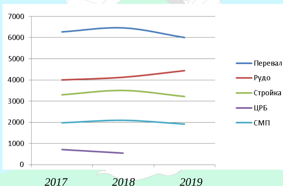
Рисунок 1.8 – Динамика планового расхода топлива «Центральной» котельной
