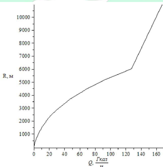
Рисунок 6.1 - График радиуса теплоснабжения для канальной прокладки
