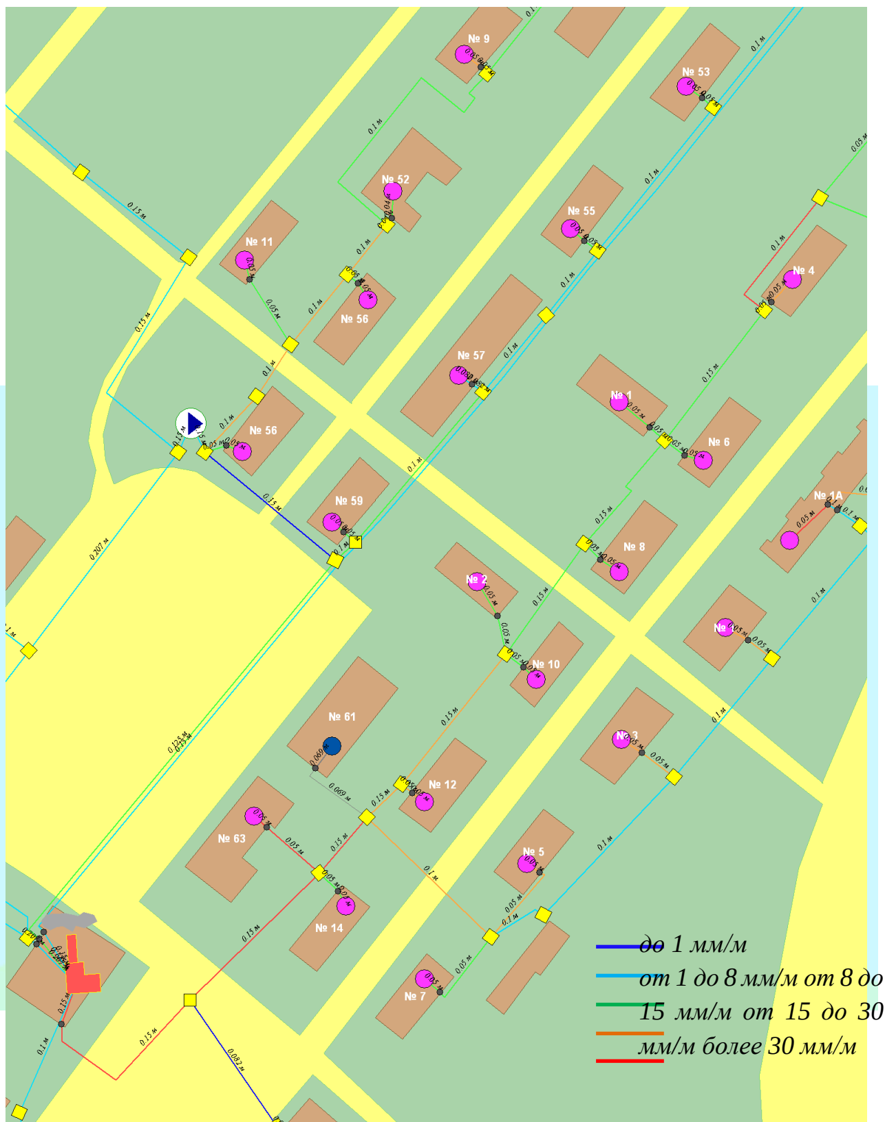
Рис.3.12 - Удельные потери по участкам теплосети от котельной Рудо
